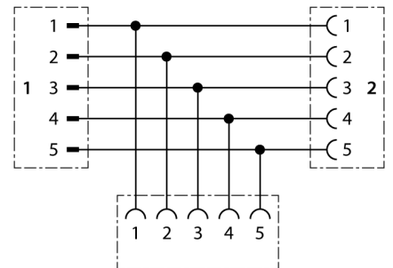
电路图
